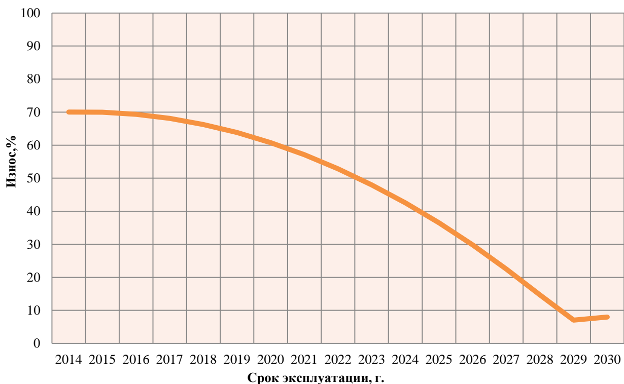
Рис. 7.2 - Зависимость износа тепловых сетей от срока эксплуатации
